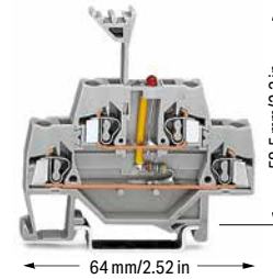
280-943/281-434 280-943/281-413
