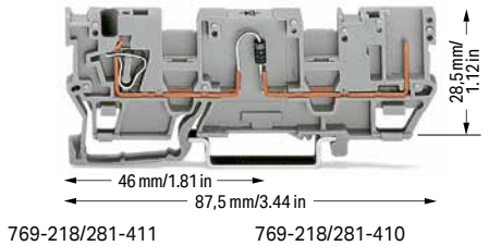
769-218/281-411 769-218/281-410
