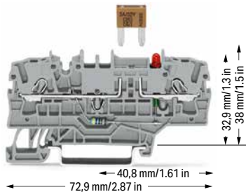
2002-1981/1000-413
