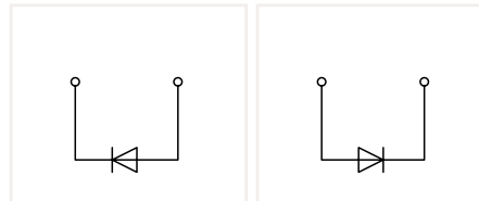
769-228/281-411 769-228/281-410
