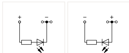
279-674/281-434 279-674/281-413
