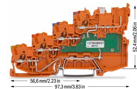
2020-5477/1102-953
