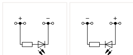
279-809/281-434 279-809/281-413
