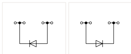
279-815/281-411 279-815/281-410
