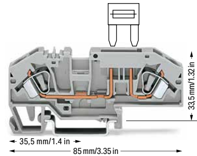
282-696
