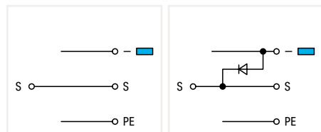
280-572 280-572/281-411
