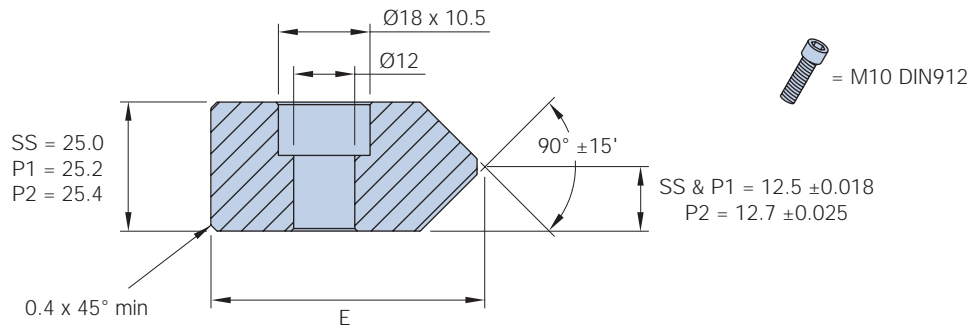
Sección X-X del anillo
